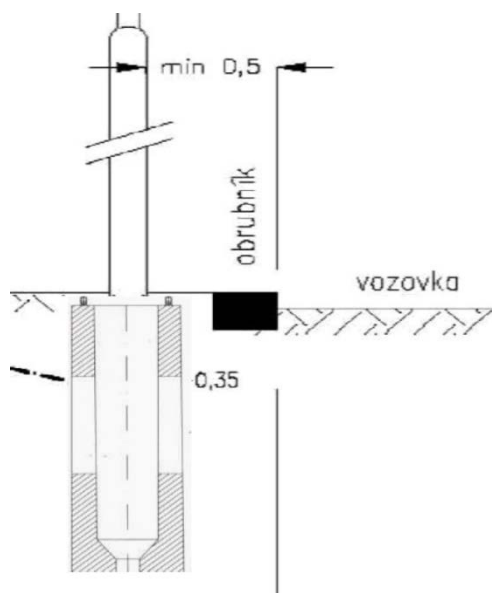
Obr. 6 - Vzorový řez vzdálenosti stožáru (patice) od komunikace.
