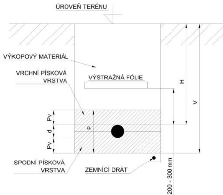
Obr. 18 - Vzorový řez uložení kabelového vedení VO s mechanickou ochranou v provedení pouze z pískového lože a s položením výstražné bezpečnostní fólie do výkopu.
