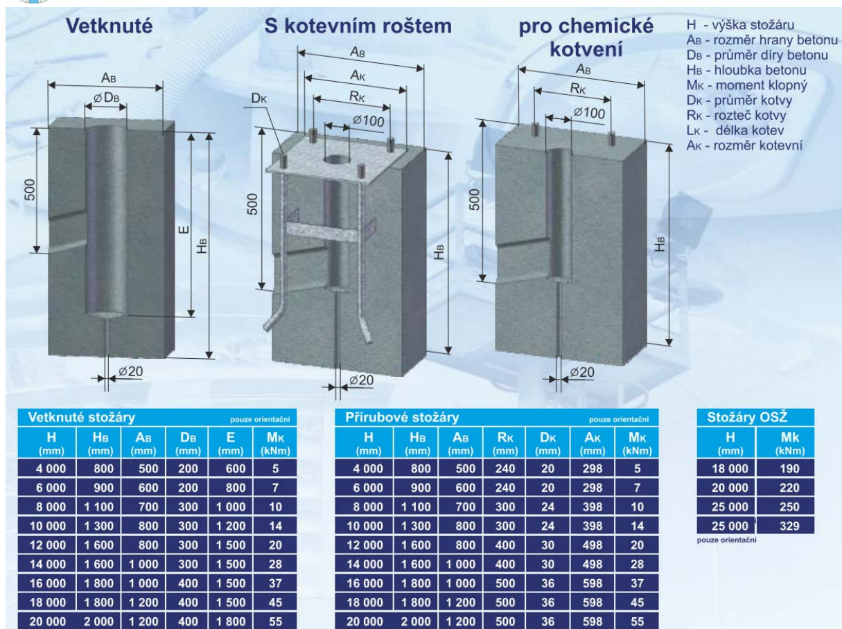
Obr. 8 - Doporučené charakteristiky základů pro kotvení stožárů (zdroj: www.kooperativa-vod.cz)
