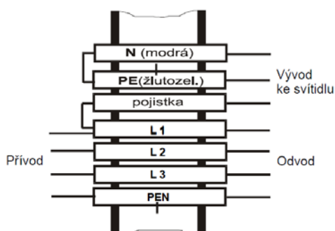
Obr. 7 - Zapojení kabelů.
