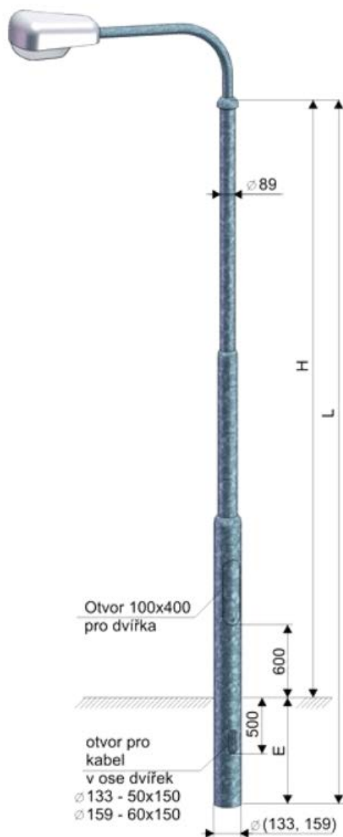
Obr. 12 - Technické specifikace stupňovité stožáry válcové pro výšku do 10 m.
