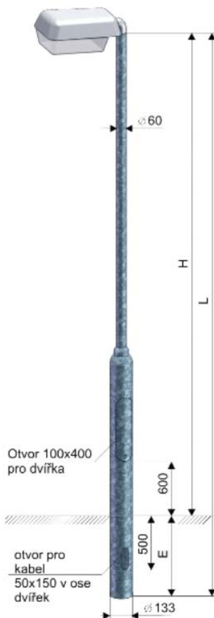
Obr. 11 - Technické specifikace stupňovité stožáry válcové pro výšku do 6 m.
