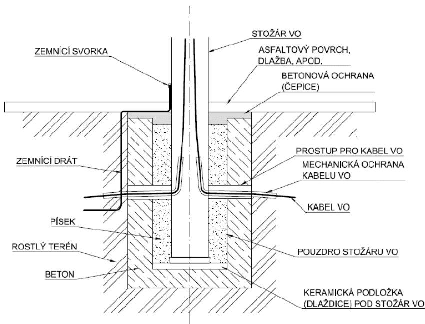
Obr. 10 - Vzorový řez základem vetknutého stožáru VO pro uložení v chodníku.
