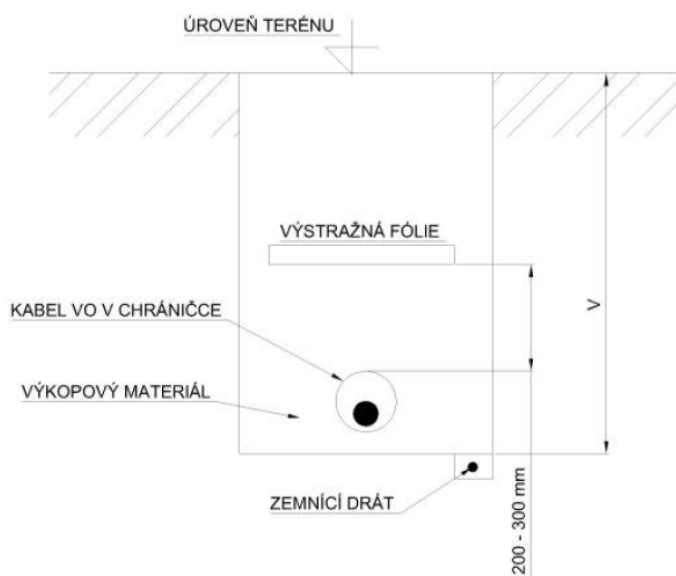
Obr. 19 - Vzorový řez uložení kabelového vedení VO s mechanickou ochranou v provedení ochranné trubky (PVC, HDPE...) a s položením výstražné bezpečnostní fólie do výkopu.
