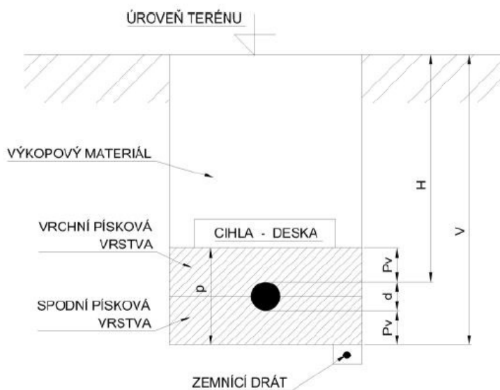
Obr. 17 - Vzorový řez uložení kabelového vedení VO s mechanickou ochranou v provedení pískové lože + mechanická ochrana nad kabelovým vedením (cihla, tvárnice, dlaždice či PVC deska).
